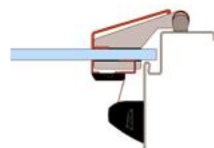
Absicherungsbeispiel NR-32 UniSafe® GLAS mit BSG 2
